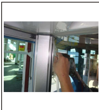
38. Klipp till den elastiska gummipackningen i rätt längd, pressa den in mellan glas och aluminiumram från toppen till botten i alla övergångar mellan glas och aluminiumram.
