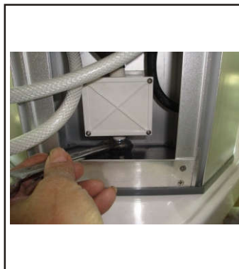
7. Skruvar och muttrar (M6x25)
